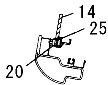
断面 Section E-E
