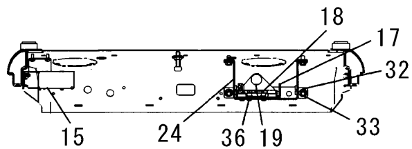
断面 Section A-A
