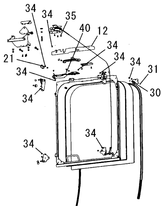
フロントガラス詳細 Detail Of Front Glass
