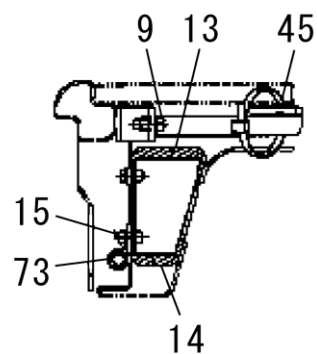
断面 Section C-C
