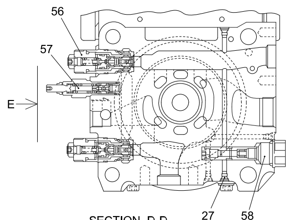
SECTION D-D
