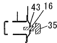
断面 Section B-B
