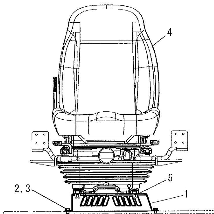
正面図 Front View
